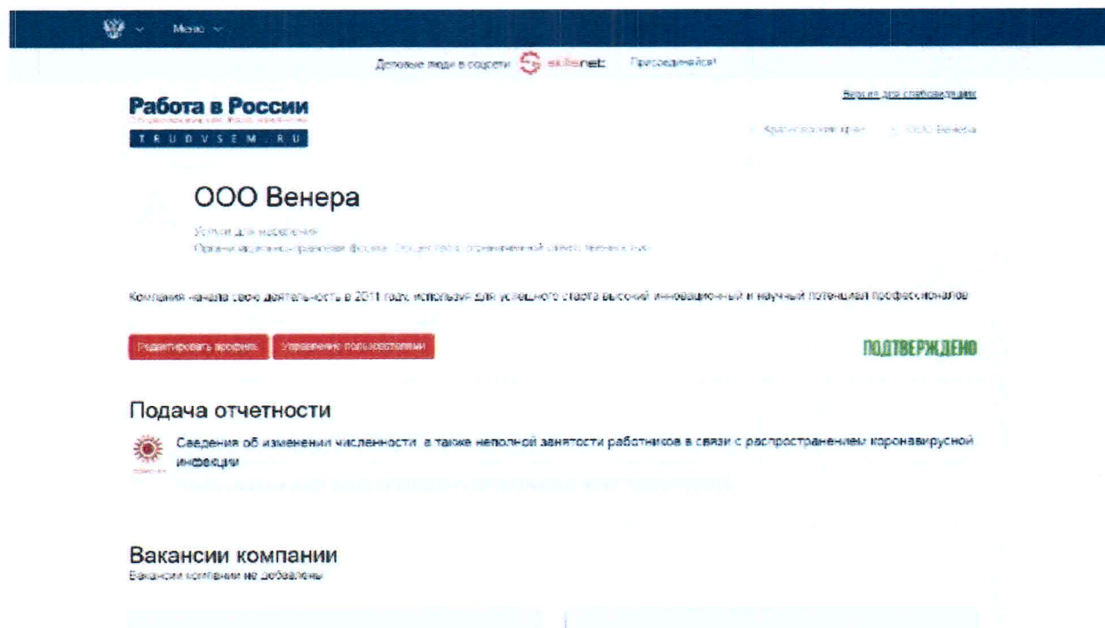
Рис. 3. Карточка компании
